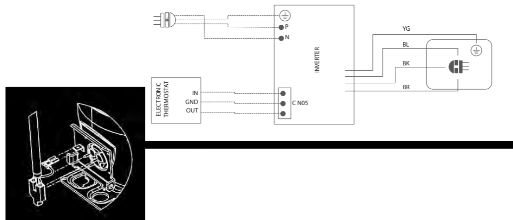
CON03 - VEMY6 / VEG (Seriale)
